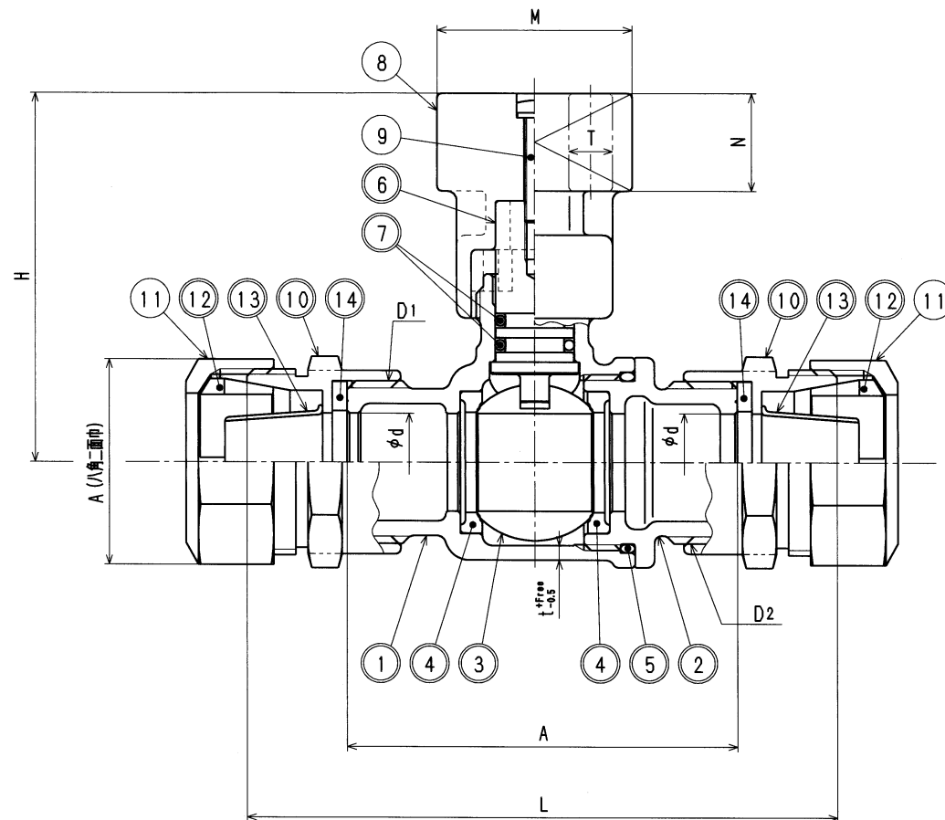
寸法表
